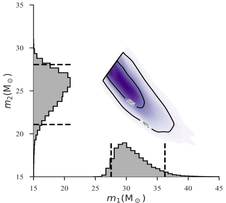
Rysunek 4: (górnny panel rysunku 4 w publikacji): pomiar mas (w masach Słońca) czarnych dziur będących składnikami układu podwójnego GW170814. Masy te są wyznaczone równocześnie z danych, dlatego ich wspólne ograniczenia są przedstawione na jednym wykresie m_2 vs. m_1 ( m_2 \leq m_1 ): im ciemniejszy kolor, tym wyższe prawdopodobieństwo, że masy czarnych dziur równają się ( m_1, m_2 ). Czarne kontury oznaczają 50% i 90% obszary wiarygodności. Dodatkowe, jednowymiarowe rozkłady prawdopodobieństwa indywidualnych mas są zaznaczone kolorem szarym.
